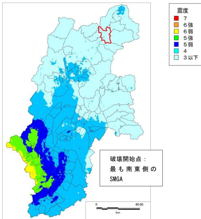
(図1-9) 阿寺断層帯(主部南部) の地震(Mj7.8)の地表震度分布
