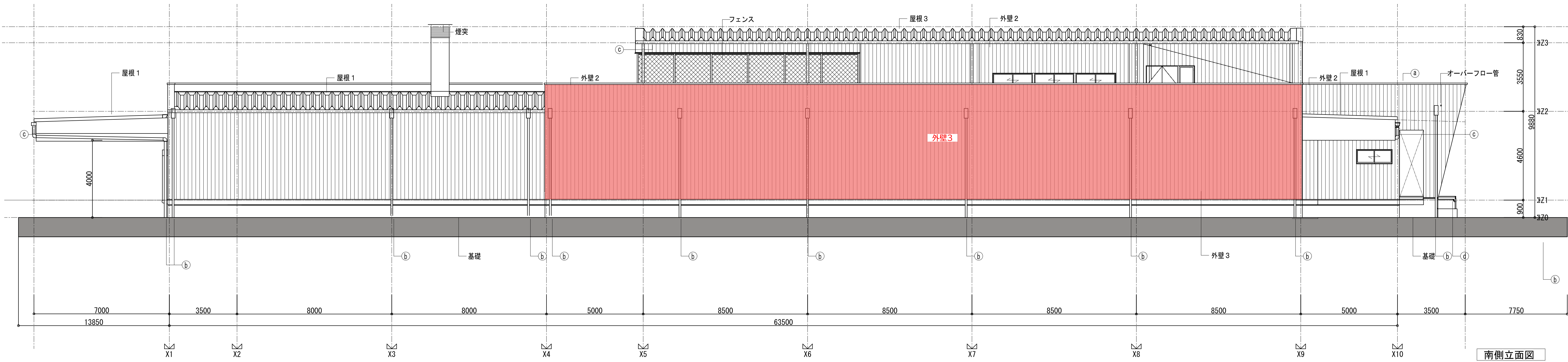
南側立面図
