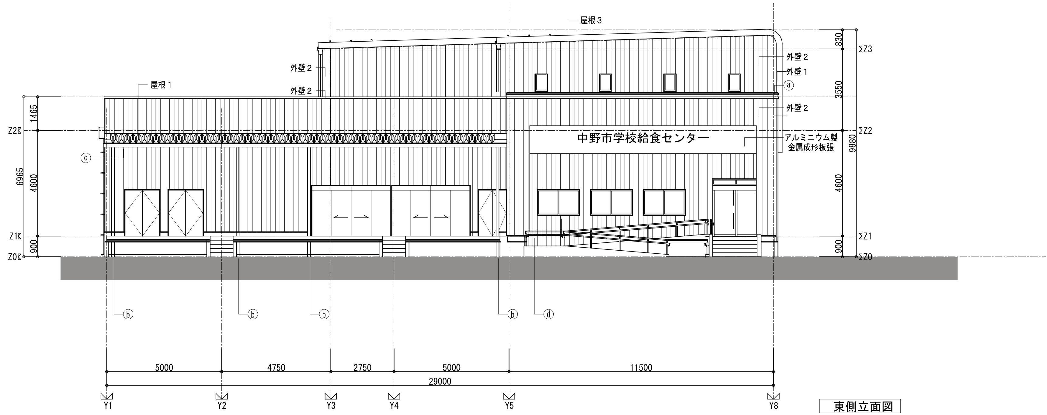
東側立面図
