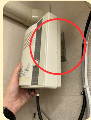
③ 端末機を上にもずらすと掛時計のように外れます。
